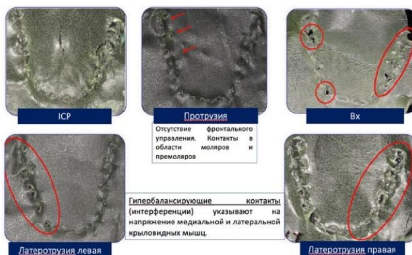
Рис.4. Окклюзиограммы пациентов.
